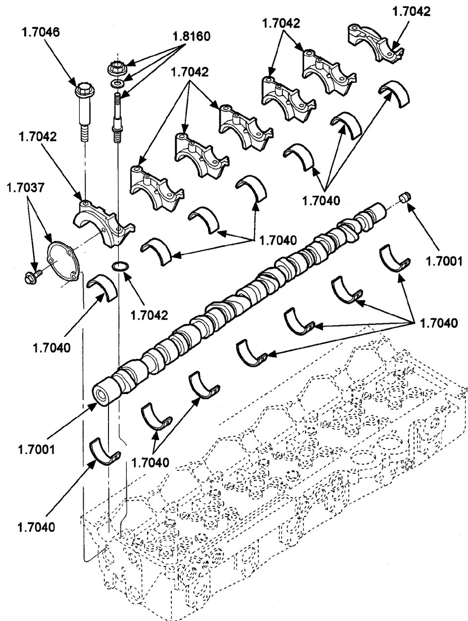
FIG. 1 CAMSHAFT
