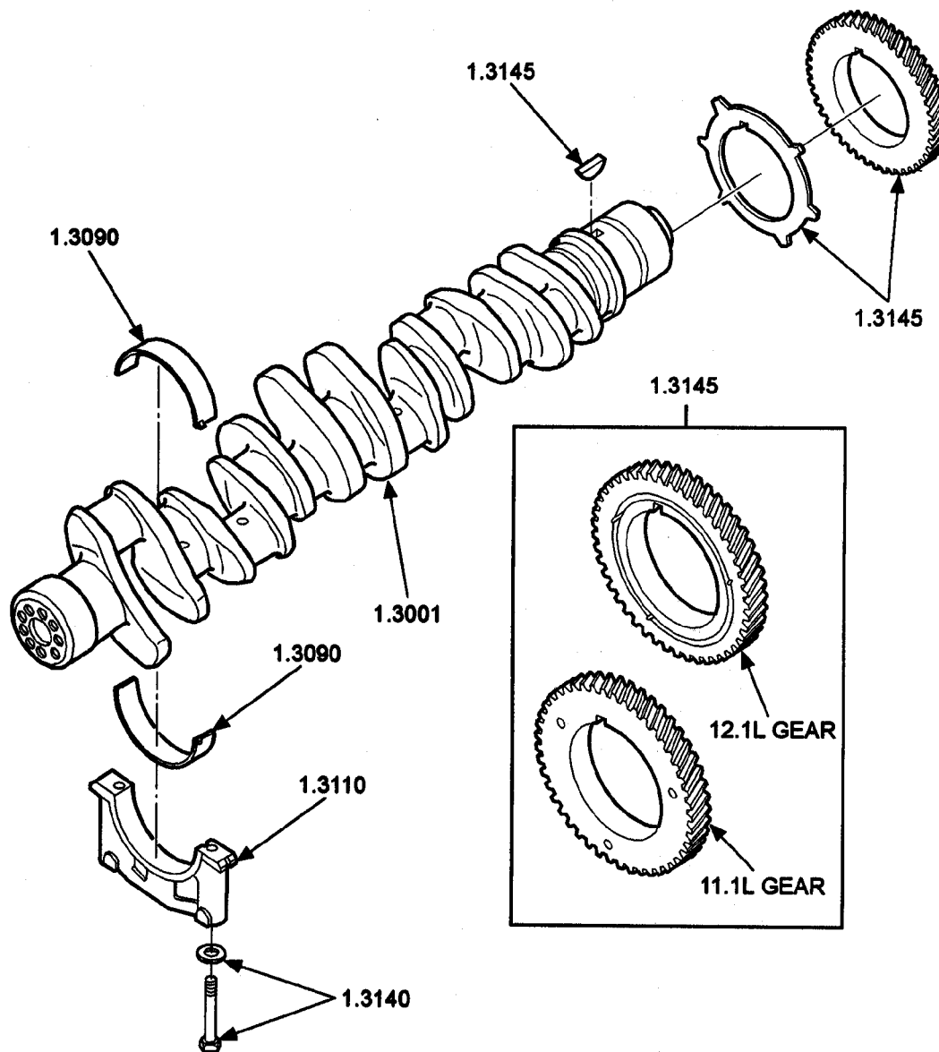
FIG. 1 CRANKSHAFT
